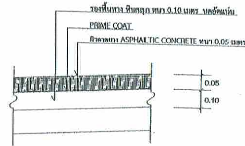
รูปตัดตามขวาง
