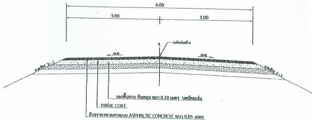
รูปตัดแสดงโครงสร้างถนน และคุณสมบัติวัสดุ(ช่วงที่ 1)
